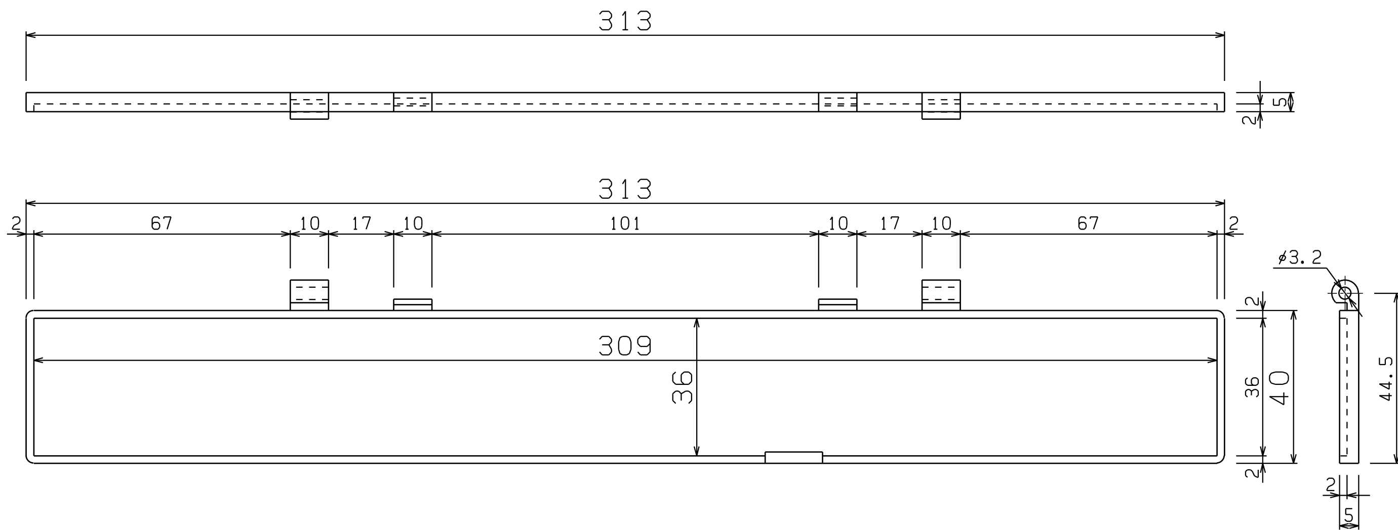
CP-108・CP-208用 フラップ
